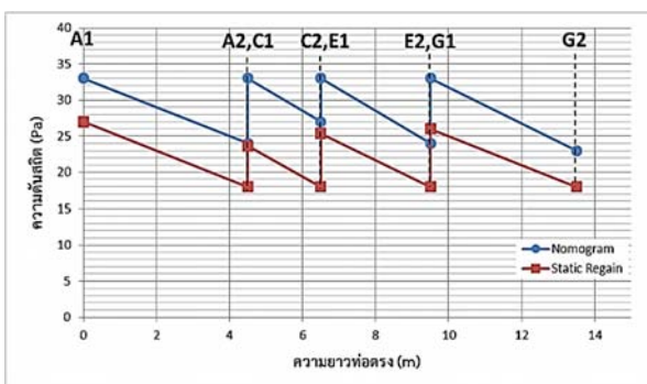
รูปที่ 15 การกระจายของความดันสถิตตามแนวความยาวของท่อตรง A,C,E,G (เลข 1 และ 2 ใช้แสดงตำแหน่งขาเข้าและขาออกของท่อตามลำดับ)
