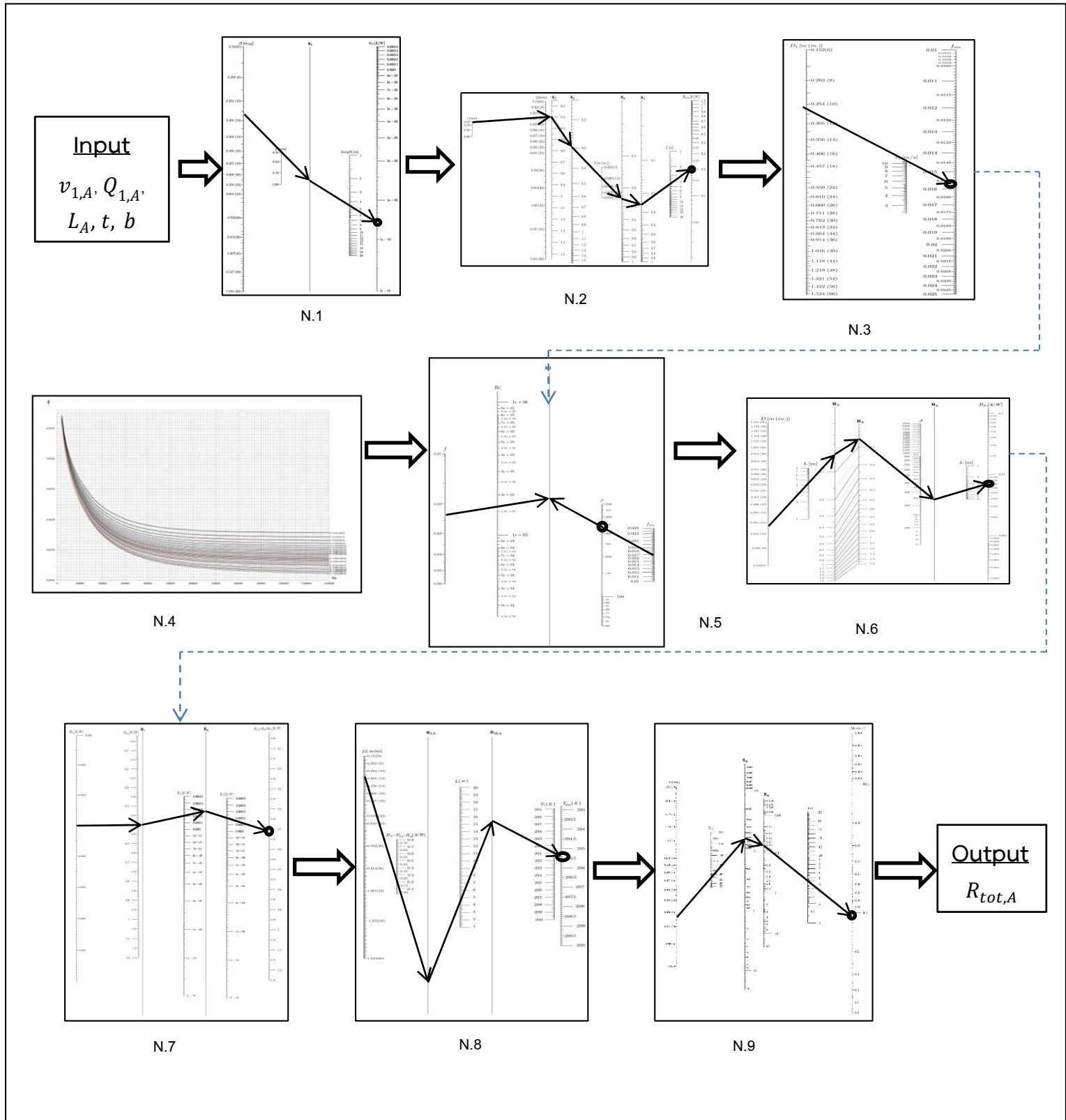
รูปที่ 6 แผนผังการใช้โปรแกรมเพื่อหาความต้านทานเชิงความร้อนรวม ( R_{tot} )
