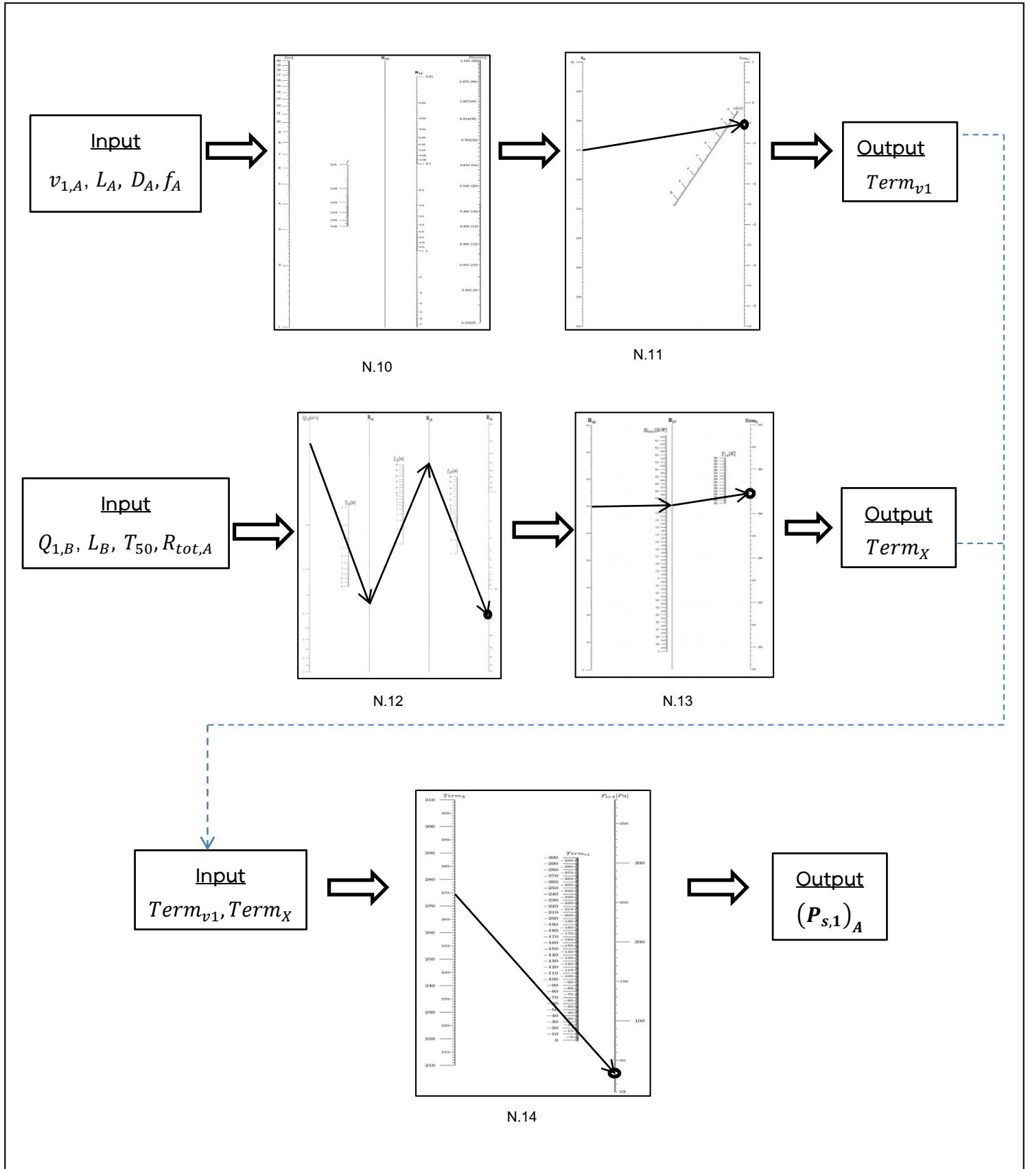
รูปที่ 7 แผนผังการใช้โนโมแกรมเพื่อหาความดันสถิตขาเข้าท่อลมท่อนแรก หรือ ความดันพัคลม (P_{s,1})_A
