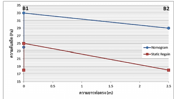
รูปที่ 16 การกระจายของความดันสถิตตามแนวความยาวของท่อ B (เลข 1 และ 2 ใช้แสดงตำแหน่งขาเข้าและขาออกของท่อตามลำดับ)
