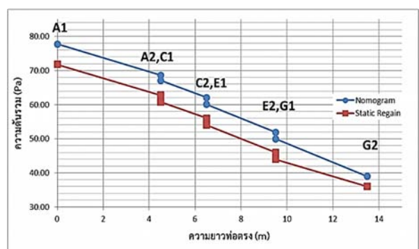
รูปที่ 17 การกระจายของความดันรวมตามแนวความยาวของท่อตรง A,C,E,G (เลข 1 และ 2 ใช้แสดงตำแหน่งขาเข้าและขาออกของท่อตามลำดับ)
