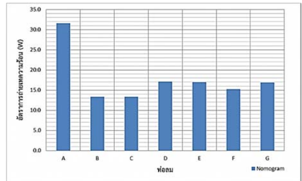
รูปที่ 19 อัตราการถ่ายเทความร้อนของท่อลม
