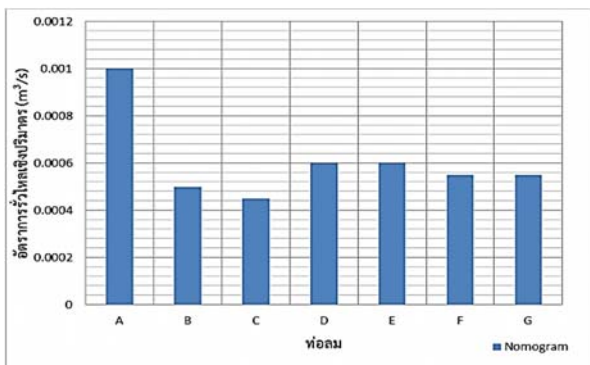
รูปที่ 18 อัตราการรั่วไหลเชิงปริมาตรของท่อลม ตารางที่ 6 อัตราส่วนความดันสถิตลดในท่อต่อความยาวของท่อลมแต่ละท่อน
