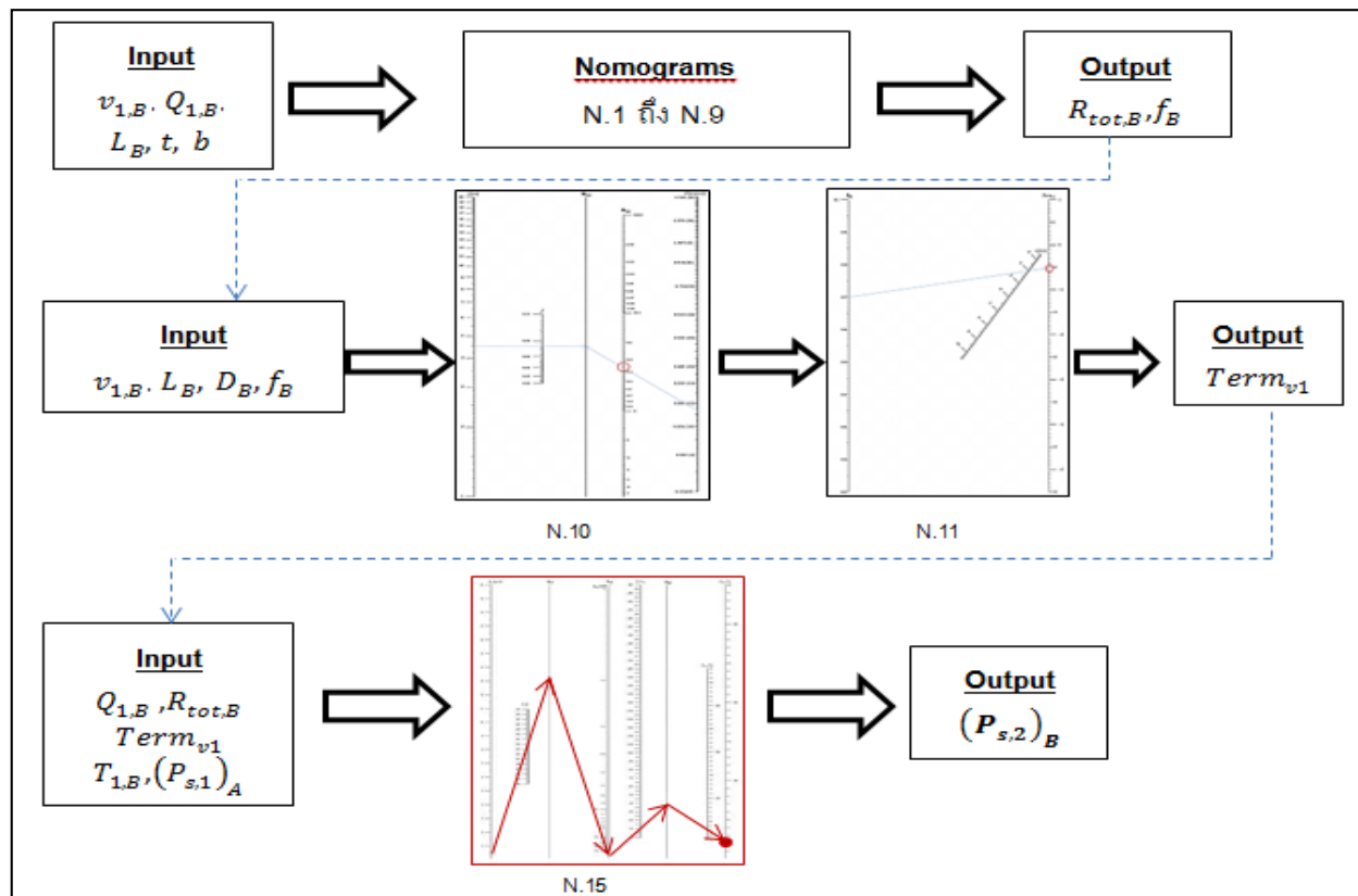
รูปที่ 13 แผนผังการใช้โนโมแกรมเพื่อหาความดันสถิตขาออกท่อสาขา ( (P_{s,2})_B )
