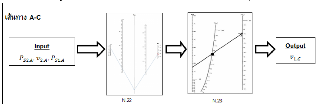
รูปที่ 12 แผนผังการใช้โนโมแกรมเพื่อหาความเร็วขาเข้าท่อตรงท่อนัดไป ( v_{1,C} )
